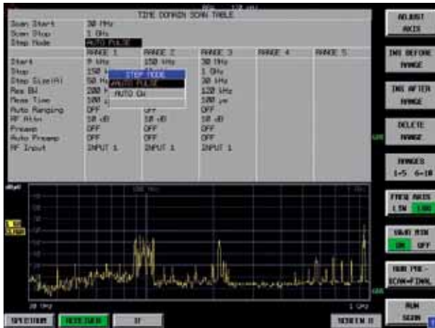
使用扫描列表编辑器进行快速时域扫描(FFT)
